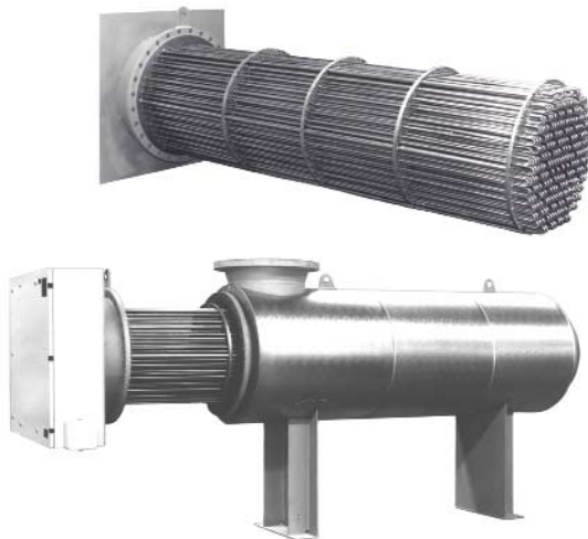
Regeneriergaserhitzer 790 kW, 350 °C, 3,75 bar Regeneration gas heater 790 kW, 350 °C, 3,75 barg
